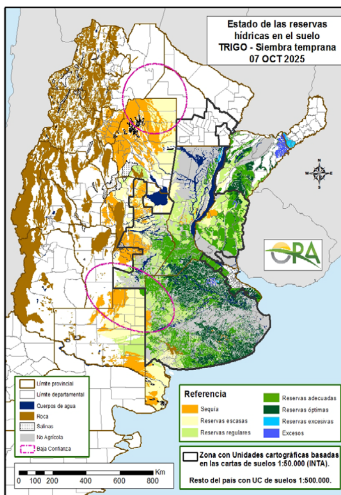
Mapa de reservas hídricas hecho a partir de datos meteorológicos del SMN y de información de suelos del INTA
