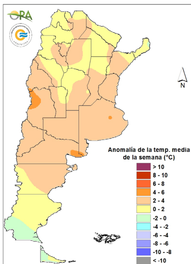
Anomalía de la temperatura media de la semana del 01/10/2025 al 07/10/2025
